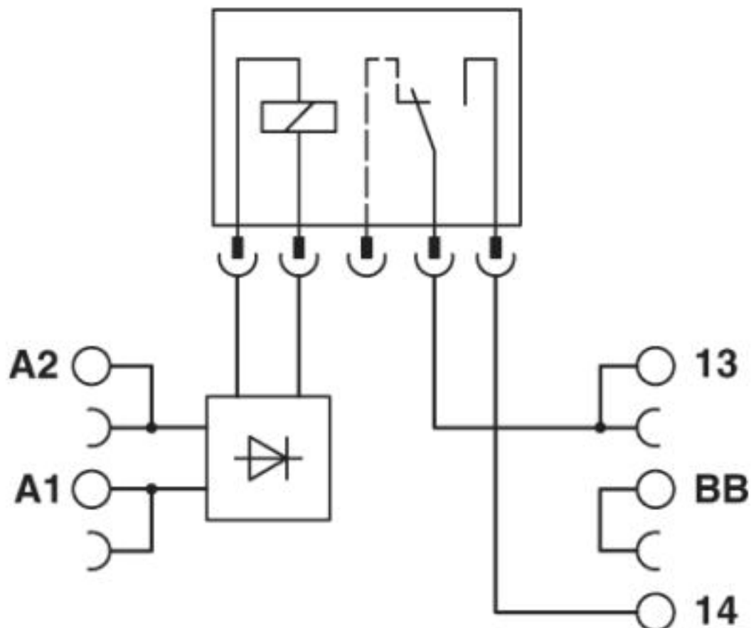
Diagrama eléctrico
